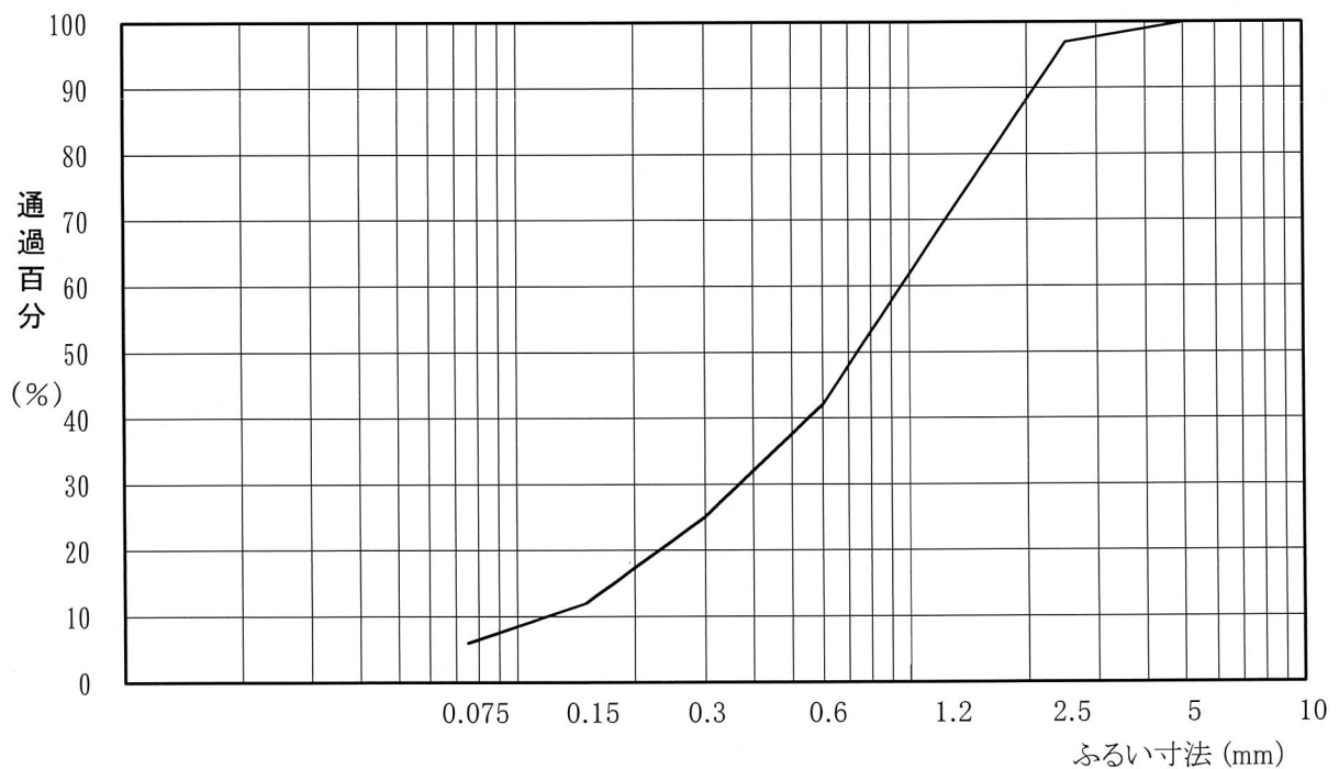
( 粒度加積曲線 )
